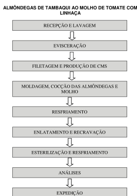
Figura 1. Fluxograma de almôndegas de tambaqui ao molho de tomate com linhaça
