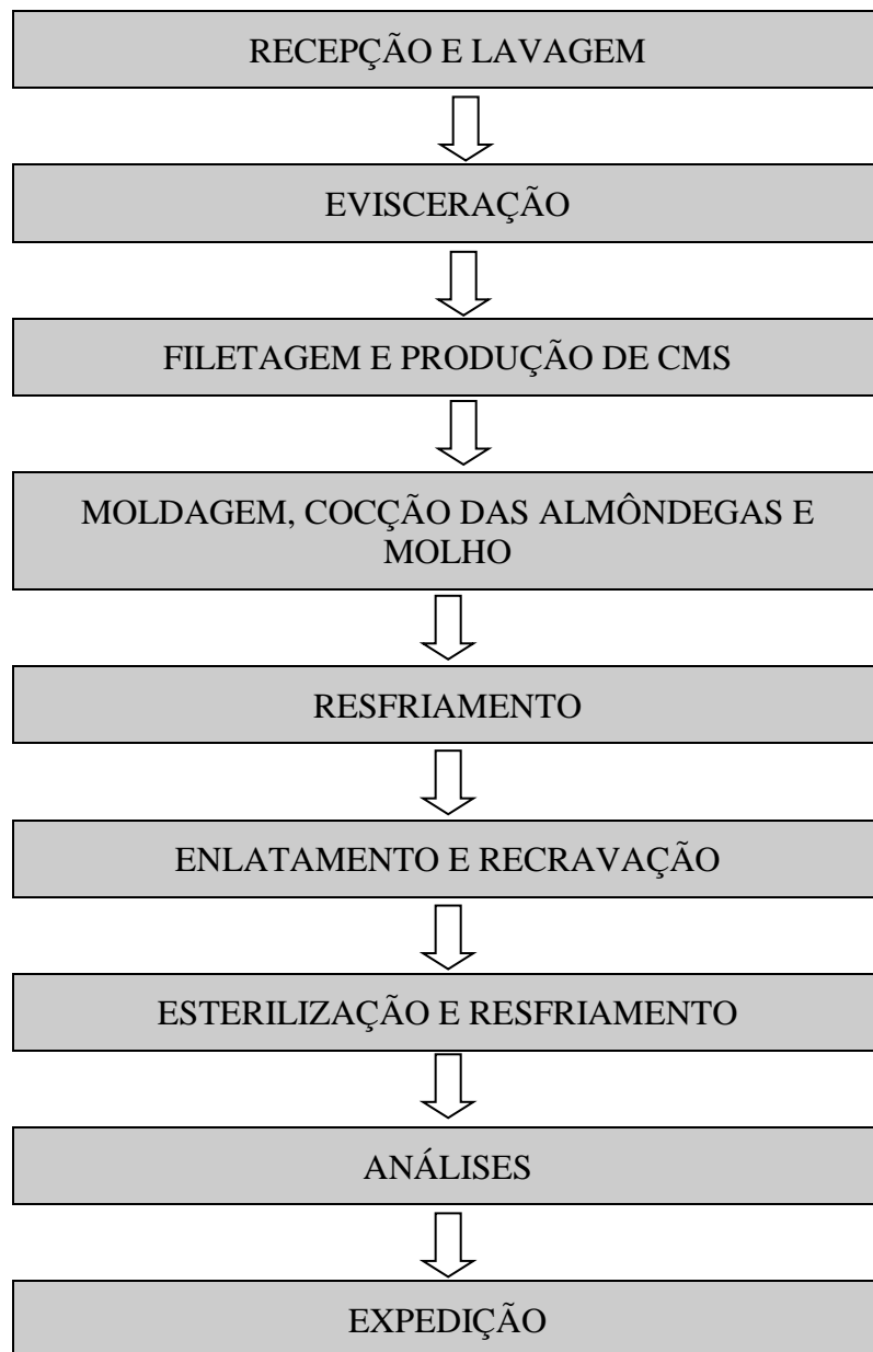
Figura 1. Fluxograma de almôndegas de tambaqui ao molho de tomate com linhaça
