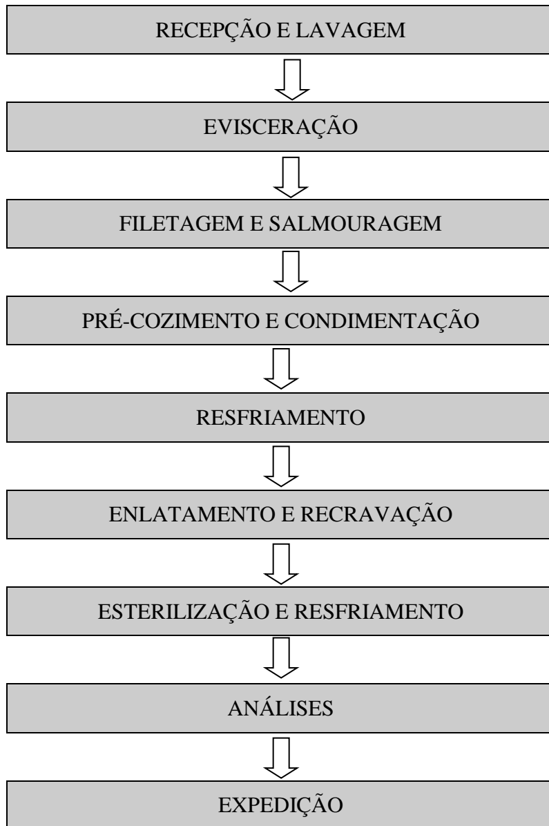
Figura 1. Fluxograma de produção de filé de pintado ao óleo comestível sabor defumado
